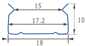
【止め金具断面図】
