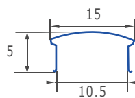
【アルミ用カバー断面図】
