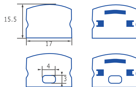
【エンドキャップ】
