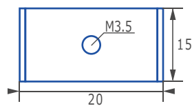
【止め金具裏部視点】
