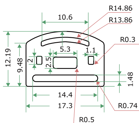
【エンドキャップ図面】
