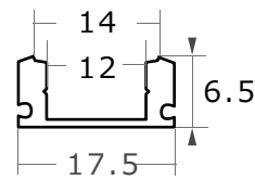
【アルミ本体断面図】
