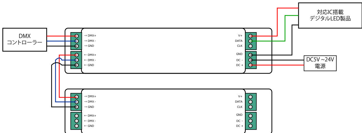
【簡易接続例】
