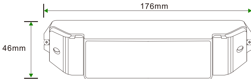
【上面図】
