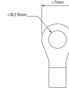
R型圧着端子
